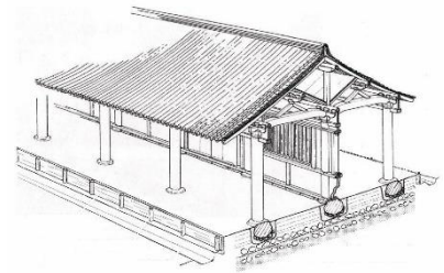
複廊の構造
