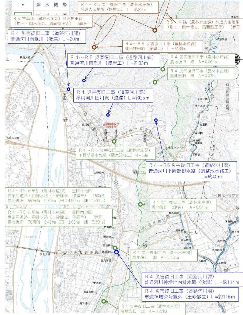
台風15号 災害復旧工事箇所図（豊岡北・南地区）【磐田市】
