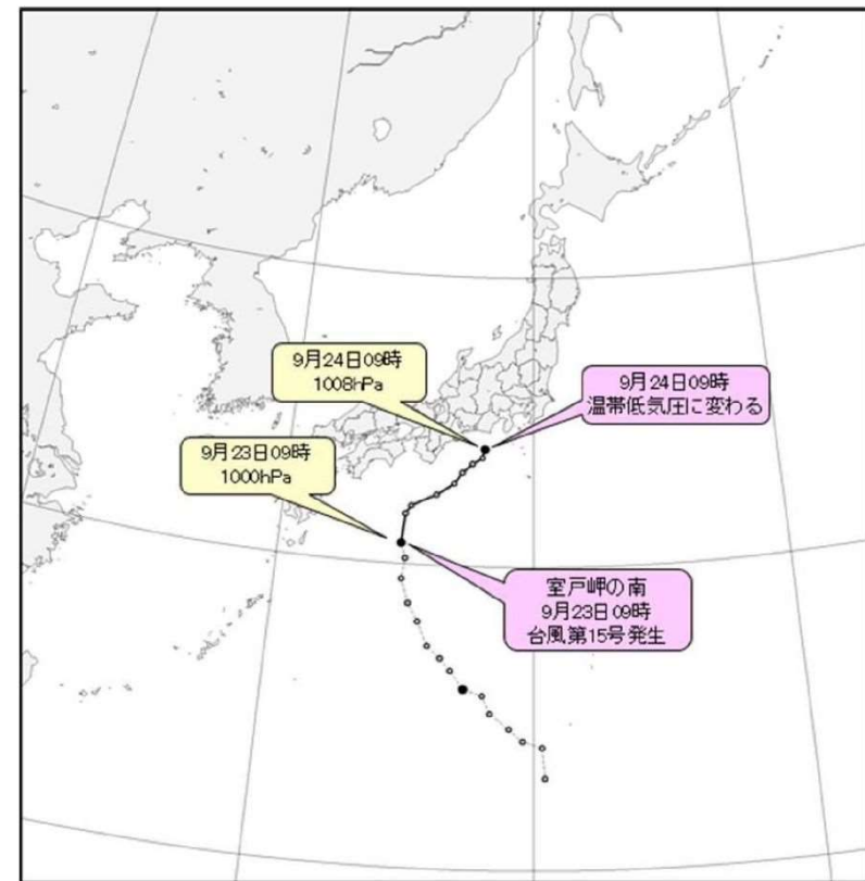
○台風経路図（日時、中心気圧（hPa））（速報解析）
