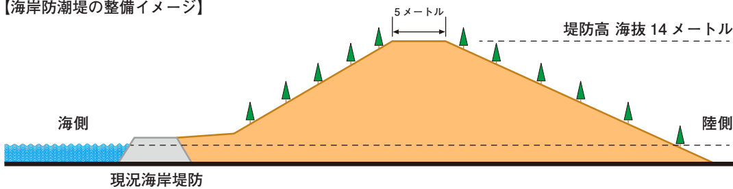
【海岸防潮堤の整備イメージ】
