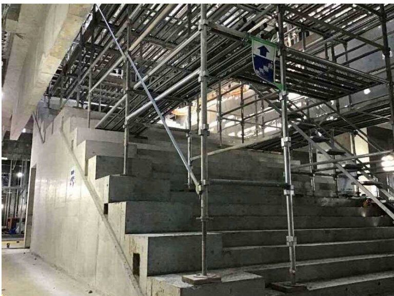
校舎棟1階 06階段3
