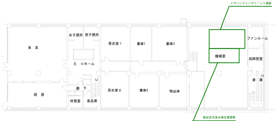
地階平面図
