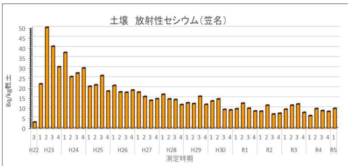
図3 土壌中の放射性セシウム濃度 (Cs-134 と Cs-137 の合計量) の経時的変化 注) 測定機関2者のうち、放射性セシウム濃度が高い値を採用している。
