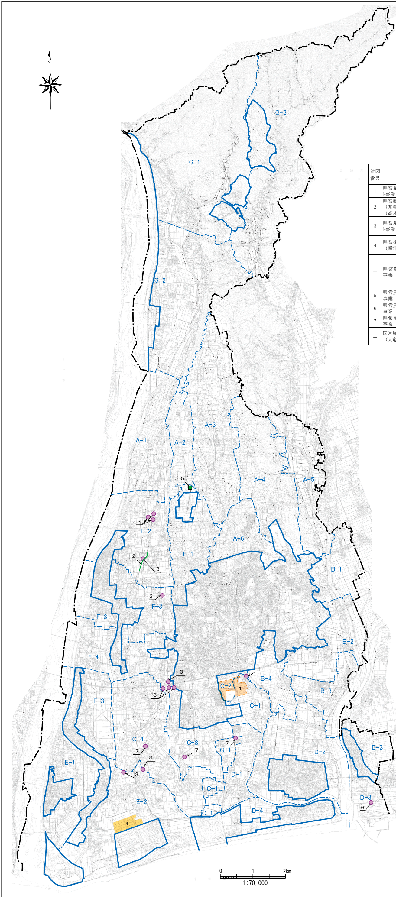
付図2号 農業生産基盤整備開発計画図
