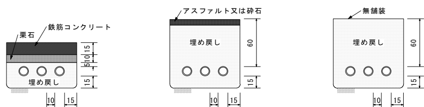
第 4－9 図 強化プラスチック製配管の埋設構造例
