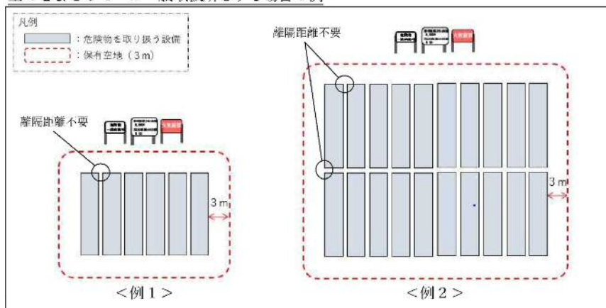
屋外コンテナ等蓄電池設備の設置例
