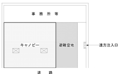
例 3 避難空地を給油取扱所の端にとらない場合
