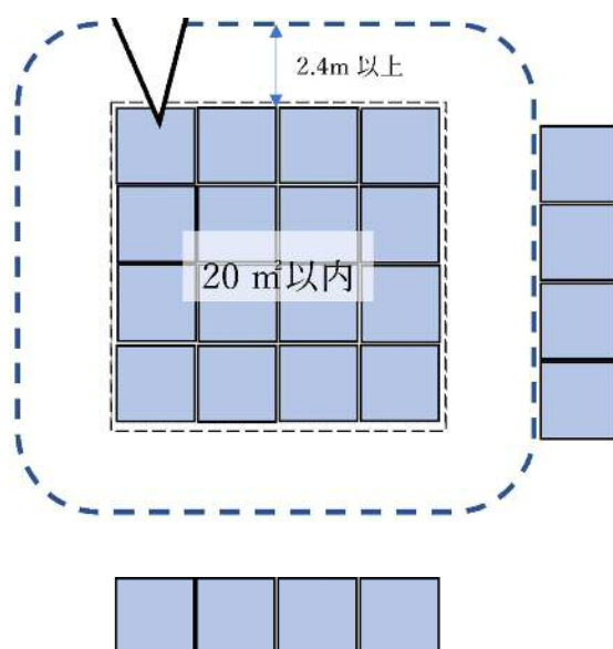
危険物の規制に関する規則第16条の2の8第2項第5号ハの貯蔵方法（例）
