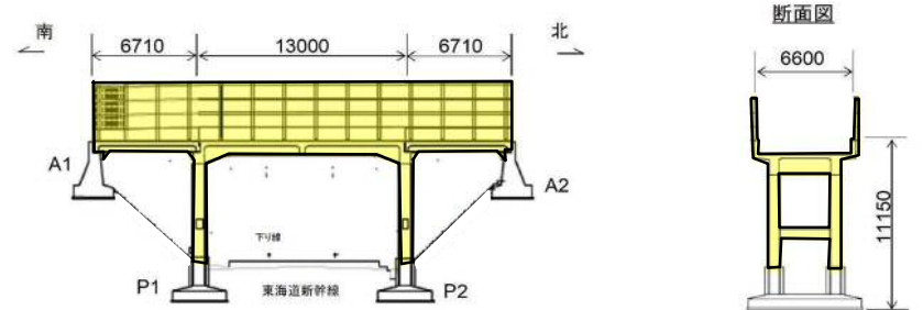
○三ヶ野新貝跨線橋 (2号橋) 竣工年度：昭和39年 構造形式：コンクリート橋
