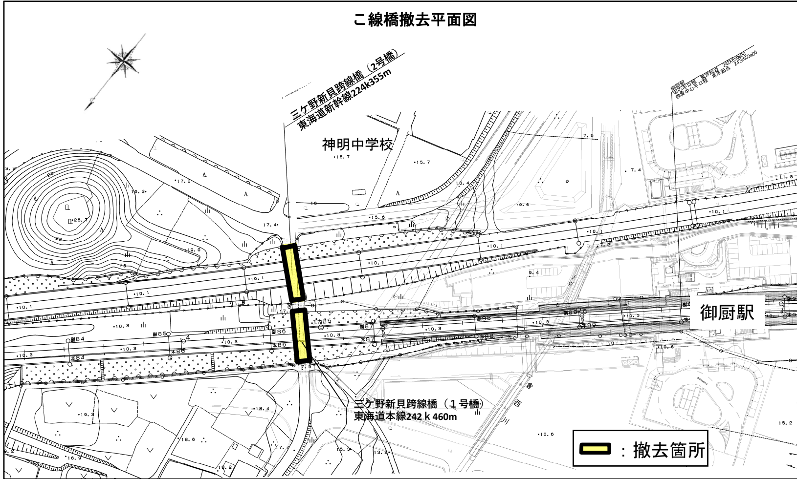
○三ヶ野新貝跨線橋 (1号橋) 竣工年度：昭和39年 構造形式：コンクリート橋
