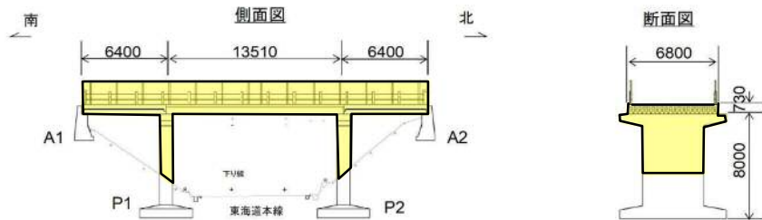
○三ヶ野新貝跨線橋 (1号橋) 竣工年度：昭和39年 構造形式：コンクリート橋
